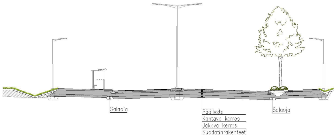
Kuva 3. Tien tyypileikkauskuvaa.
